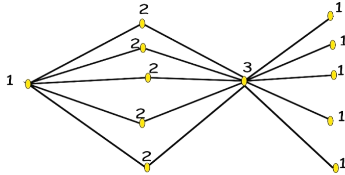
Figure1: \psi[S(K_{1,5})] = 3
